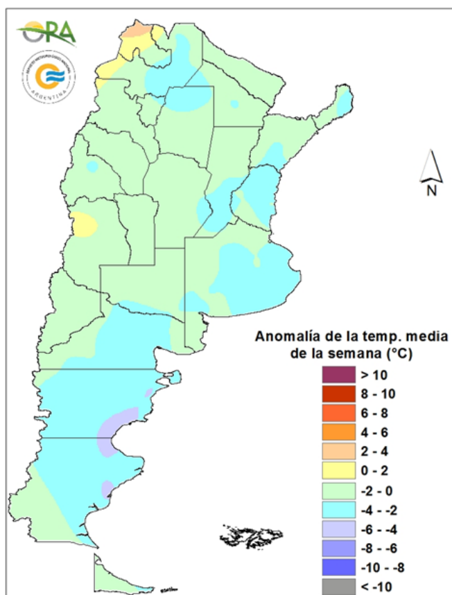
Anomalía de la temperatura media de la semana del 04/12/2024 al 10/12/2024
