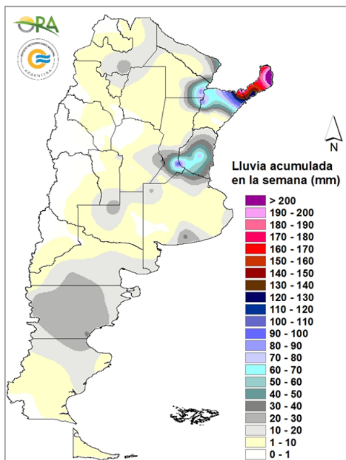
Precipitaciones acumuladas en la semana del 04/12/2024 al 10/12/2024
